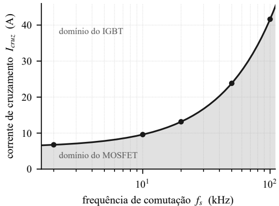
(b) V = 400\text{ V} , d = 0,5
